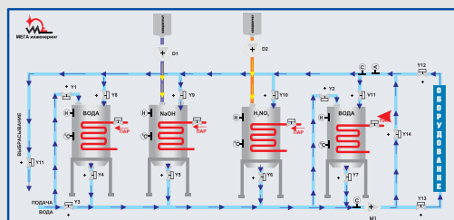
Система за контрол и управление на производствен цикъл в предприятие за млекопреработка Control and management system for the production process in dairying businesses
